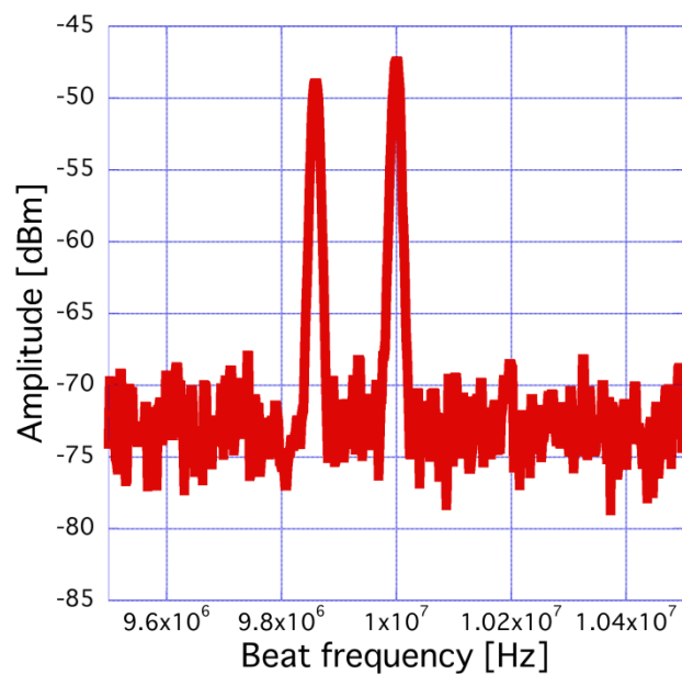
(a) 市販アンプ(帯域 100MHz)
