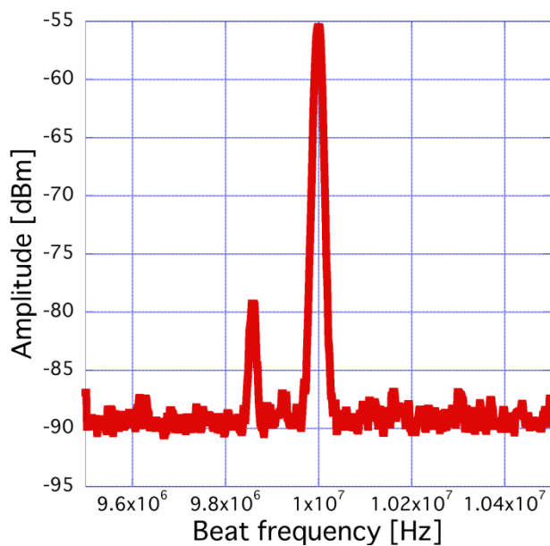
(b) AD8015
