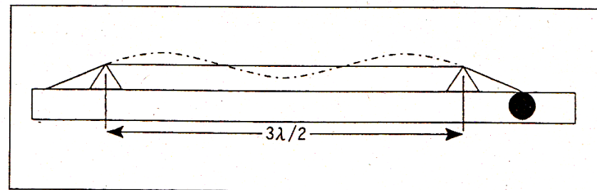
図0.32 定在波
