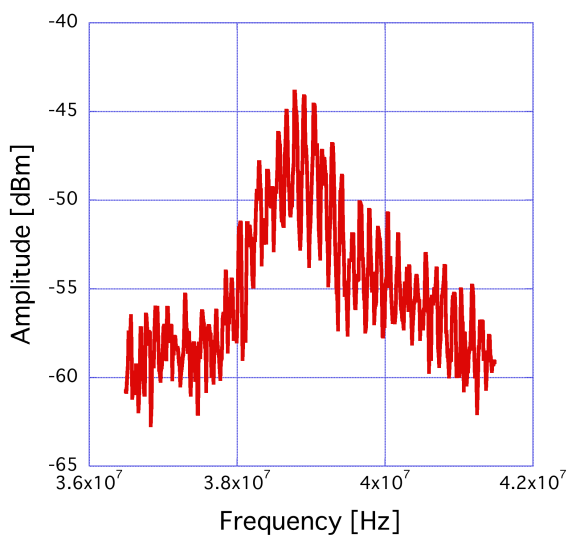
図3 40MHz 拡大図
