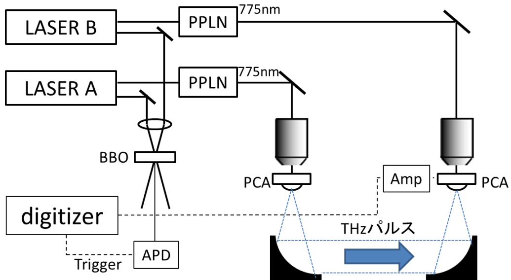
図2 実験装置
