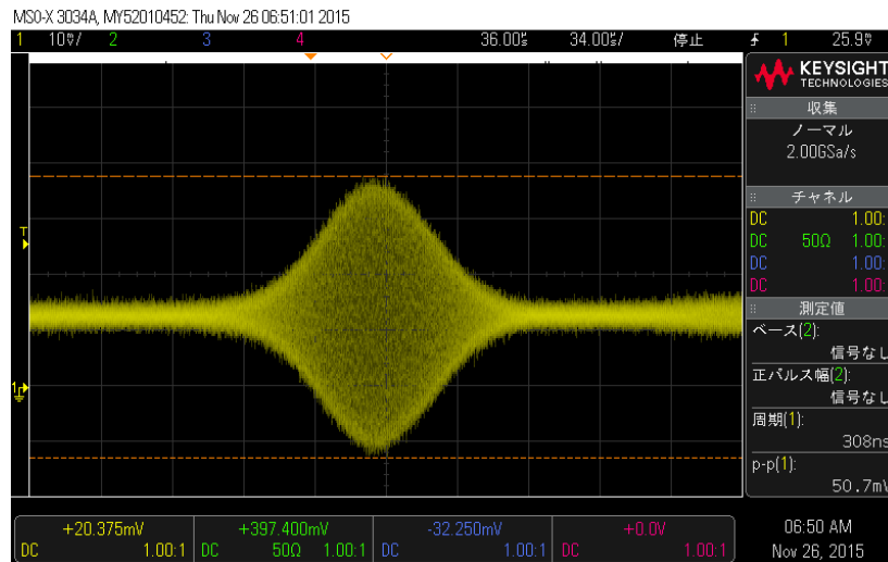
図 2 制御なしのインターフェログラム
