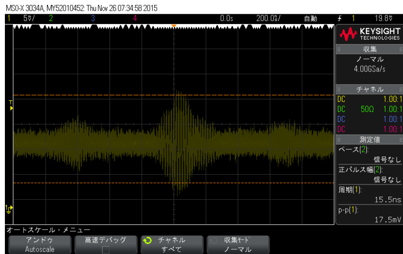
図 3 制御した時のインターフェログラム
