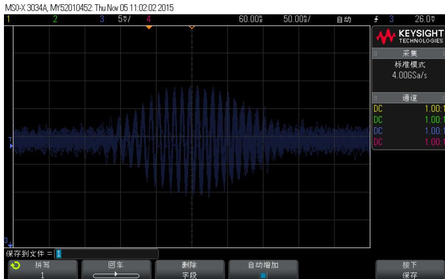
図2 取得したインターフェログラム
