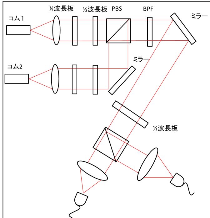
図1 デュアル光コムの光学系 (DMD なし)
