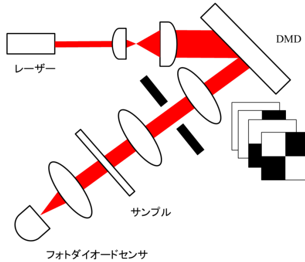
図1 光学系
