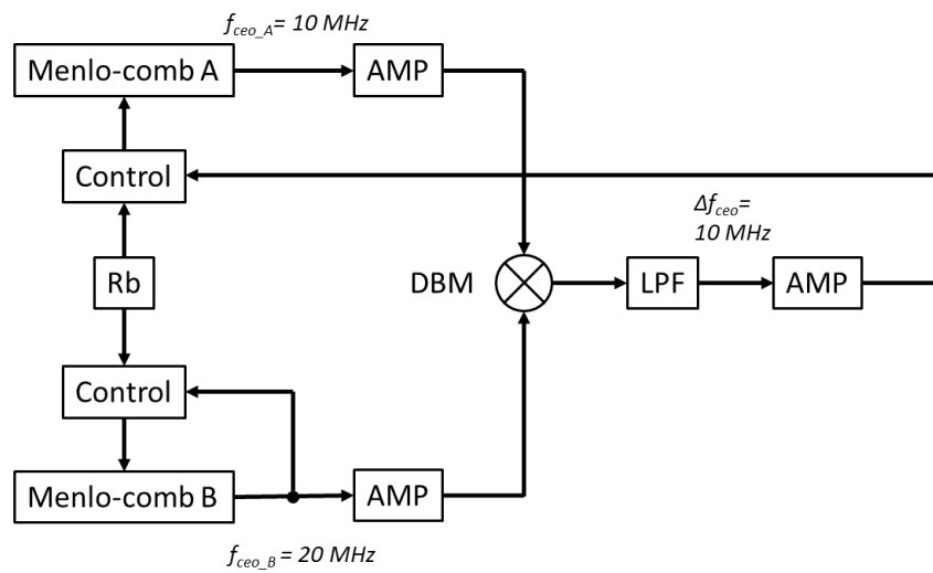
図1 制御系
