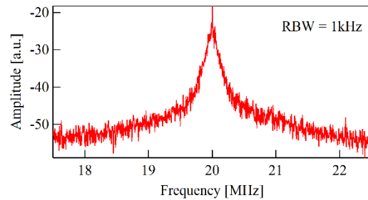
図5 f_{CEO B} (log scale)
