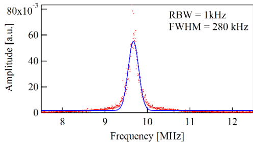
図2 f_{CEO A} (linear scale)
