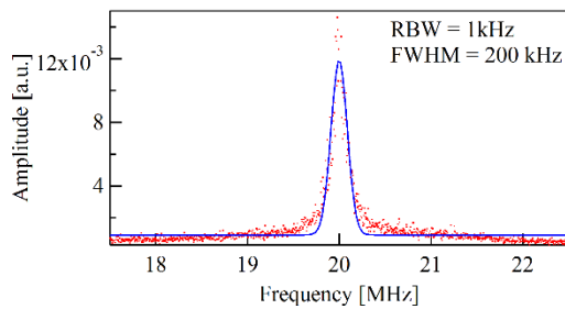
図4 f_{CEO B} (linear scale)
