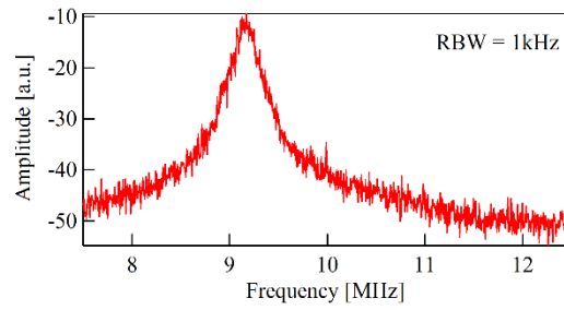
図3 f_{CEO A} (log scale)
