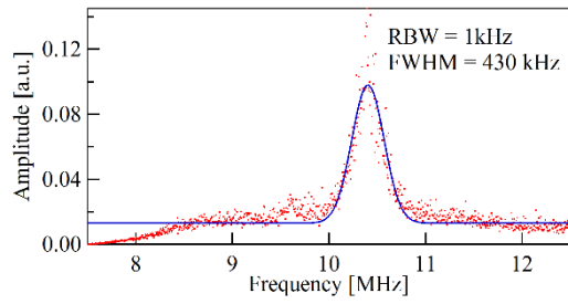
図 6 f_{CEObeat} (linear scale)
